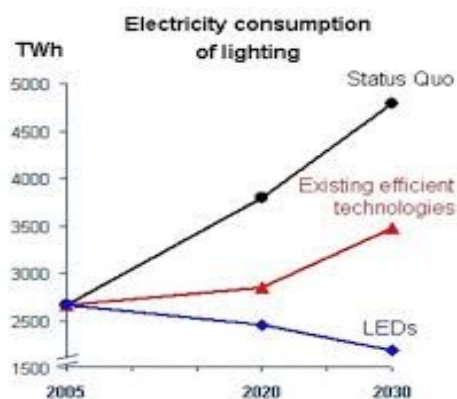
Illustratie: verwachte ontwikkeling energie gebruik LED verlichting
